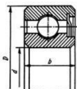
Подшипник шариковый радиальный однорядный с одной защитной шайбой
