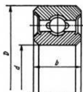
Подшипник шариковый радиальный однорядный с двумя защитными шайбами
